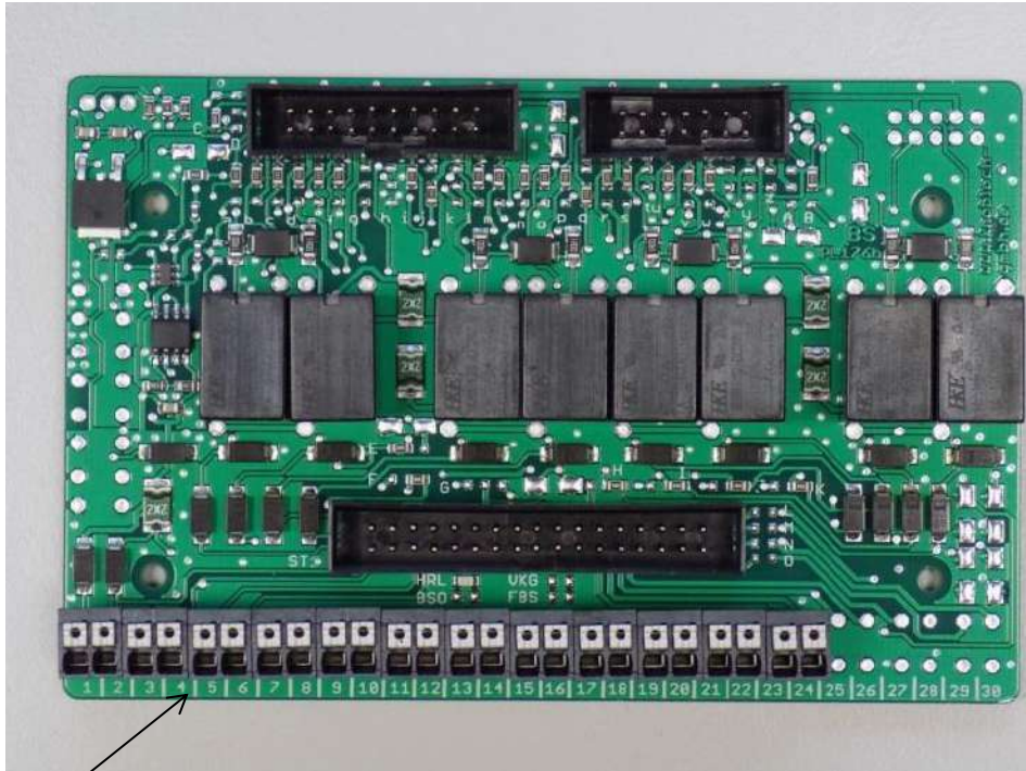
Klemmen / Terminals 1-30
